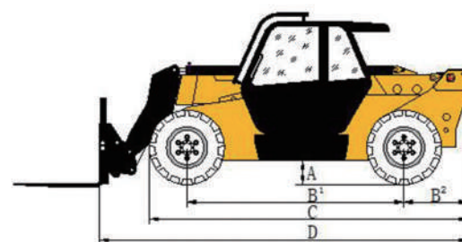
尺寸图 Dimension drawing
